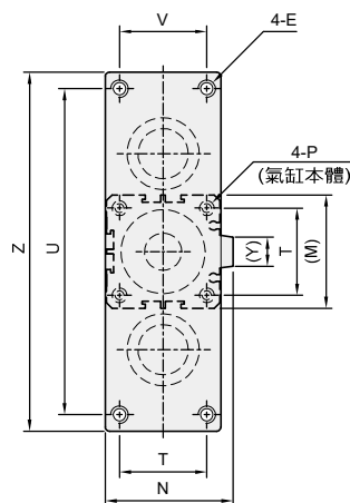
(法蘭板視圖)
