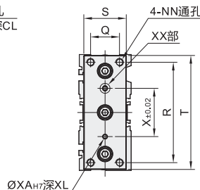
T型槽尺寸
