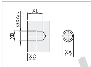
XX部详细图
