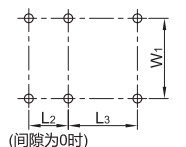
安装孔孔距
