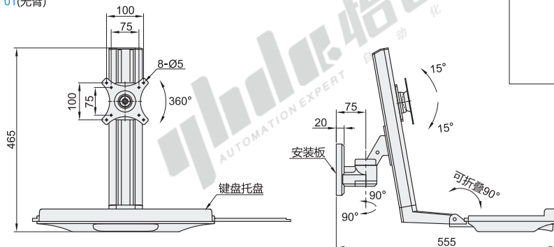
臂数: 01(无臂)
