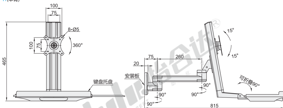
臂数: 11(单臂)
