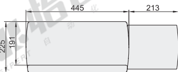
■ 键盘托盘尺寸
