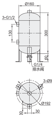
容积: 40L
