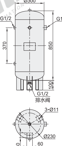
容积: 60L
