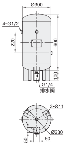
容积: 40L
