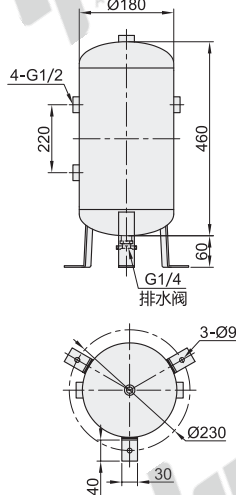
容积: 60L
