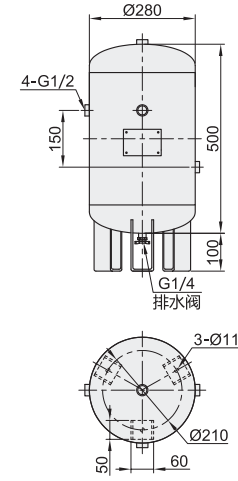
容积: 30L
