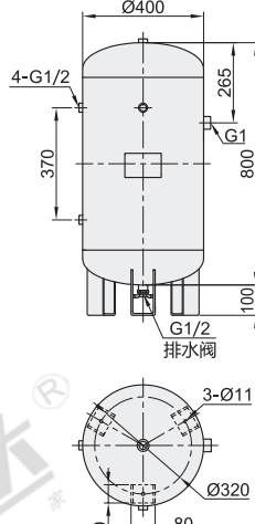
容积: 100L
