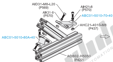
分解图
