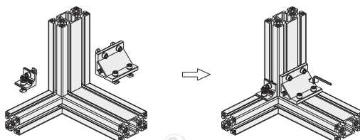
组装图
