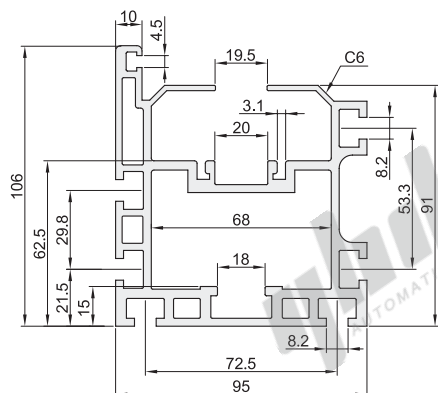
ATS05-25-38DG (此型号需另外采购钢轨)
