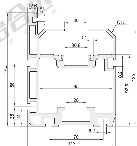
ATS05-30-50DG (此型号需另外采购钢轨)
