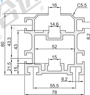
ATS05-25-31DG (此型号需另外采购钢轨)
