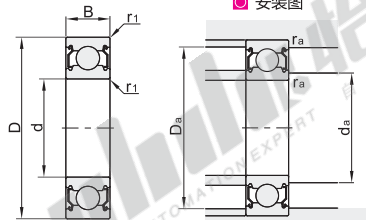
安装图
