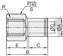
外六角直接头 XZR06
