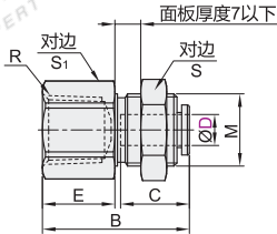
外六角隔板直接头 XZR07
