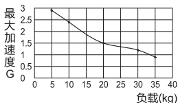
最大加速度vs负载
