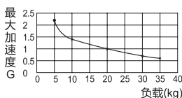
最大加速度vs负载
