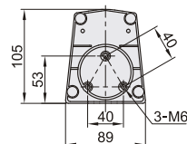
安装板尺寸
