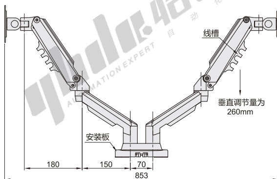
安装板尺寸
