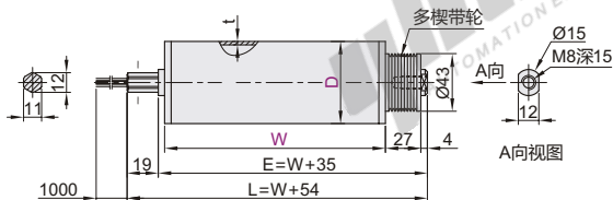
多楔带轮型 E-QCG81
