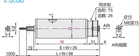
同步带轮型 E-QCG82
