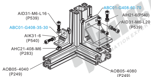
分解图
