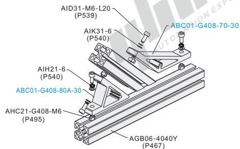
分解图
