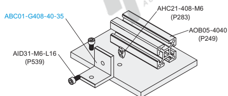
分解图
