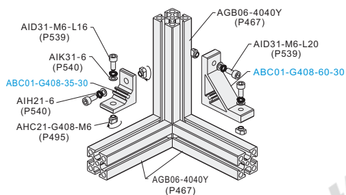
分解图
