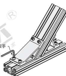
组装图
