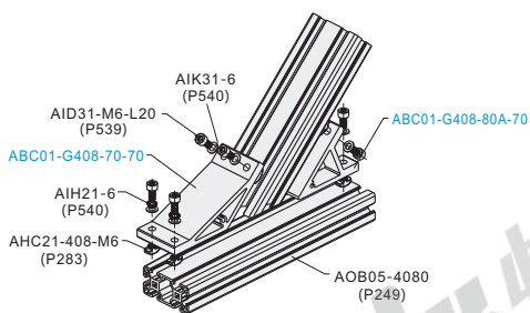
分解图
