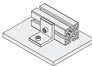
组装图
