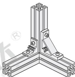
组装图
