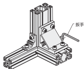
组装图
