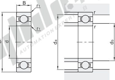
安装图
