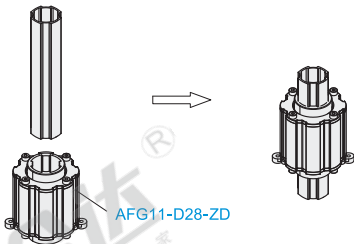
分解图
