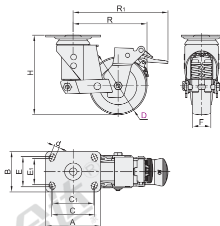
平底活动型·塑料单刹 CGL32
