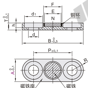
沉孔型 BMG01/06
