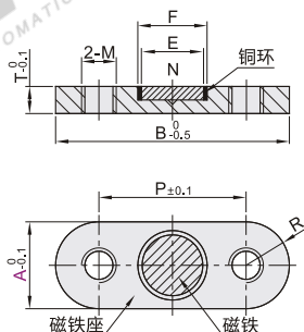
螺孔型 BMG11/16
