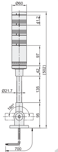
A(可折式)
