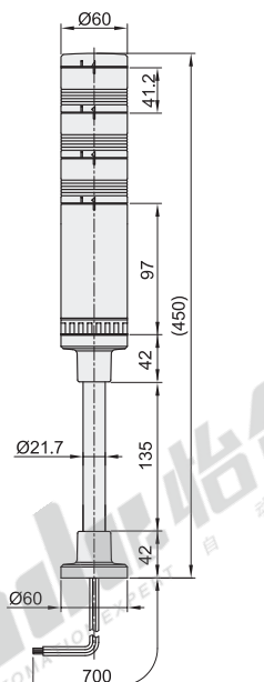
C(杆盘式)
