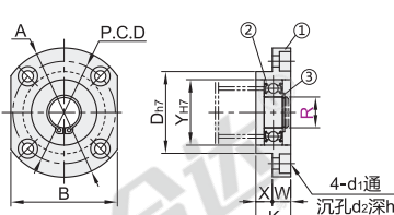
单件·支座支持侧 LHF04
