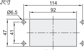
☑ 开孔尺寸
