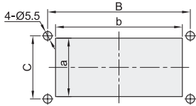
☑ 开孔尺寸
