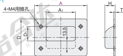
☑ 开孔尺寸
