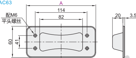
☑ 开孔尺寸
