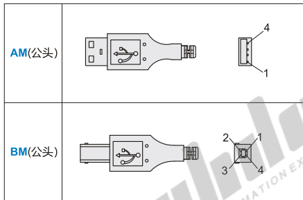
线束插头
