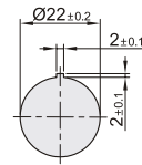
开孔尺寸
