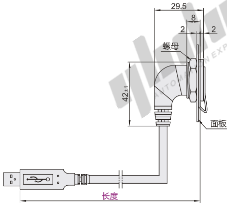
线束插头
