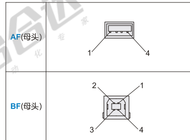
面板式插口
