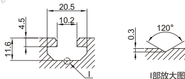
■ 槽口详图
