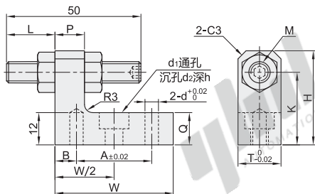
紧凑型限位块+定位螺栓
