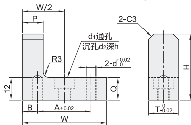
紧凑型限位块+定位螺栓
