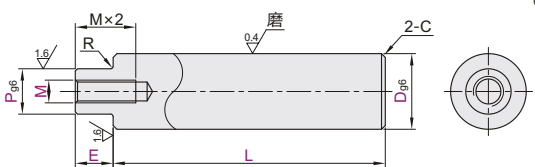
一端台阶内螺纹型 SHX21
