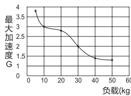
最大加速度VS负载
