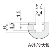
A处放大图
