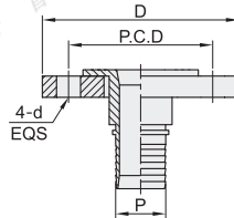
活动法兰接头 BMA03
