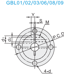
圆法兰型 GBL01/02/03/06/08/09
