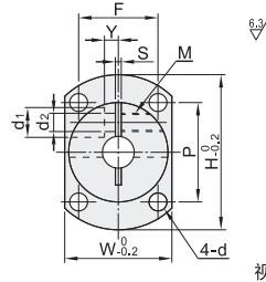
对边法兰型 GBJ21/22/23/26/28/29
