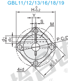
方法兰型 GBL11/12/13/16/18/19
