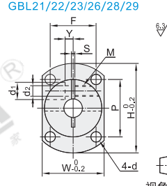
对边法兰型 GBL21/22/23/26/28/29
