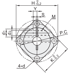
方法兰型 GBJ11/12/13/16/18/19
