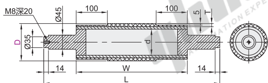
涂布压辊型 QAA71
