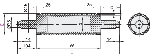
涂布牵引型 QAA76
