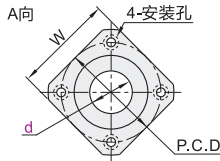
方法兰型 OFZ86
