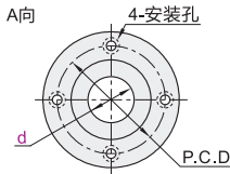
圆法兰型 OFZ81
