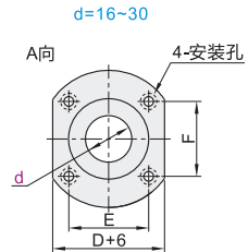
对边法兰型 OFZ91 OFZ96
