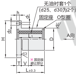
圆法兰型 OFZ81
