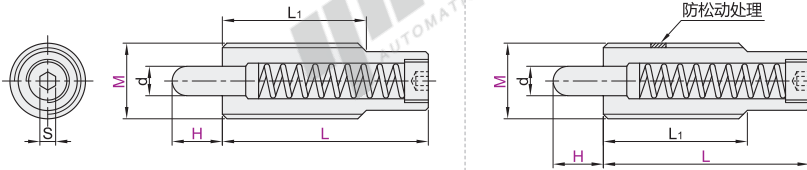
无防松型 ZAX45
