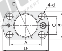
安装图
