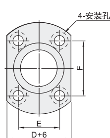
对边法兰型 d=16~50
