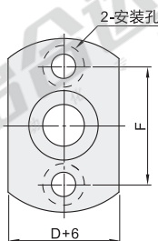
对边法兰型 d=8~13
