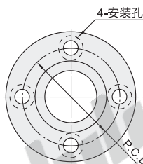
圆法兰型 d=16~50
