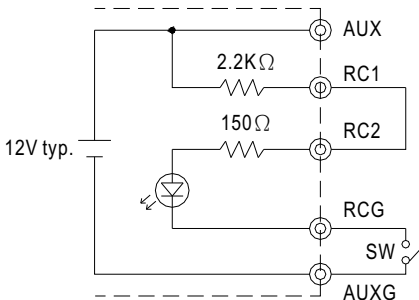
(B)使用内部12V辅助输出
