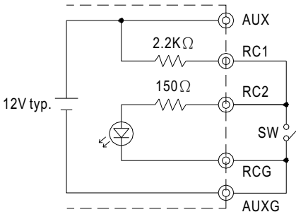
(C)使用内部12V辅助输出
