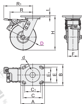
平底活动型·五金双刹 CGL35
