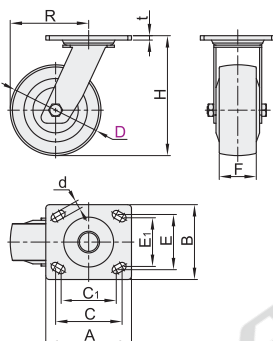
平底活动型·无刹 CGL34
