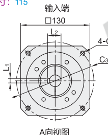
A向视图
