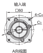
A向视图
