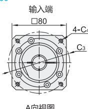
A向视图
