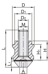
定位拉钉 ZFH63
