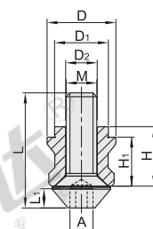
夹紧拉钉 ZFH65
