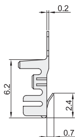
端头 ZKY27
