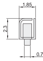
截面C-C
