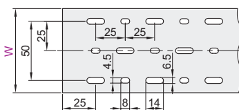
□ W≥80mm线槽底部孔尺寸
