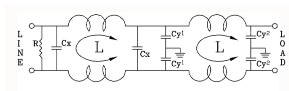
电气方案9
