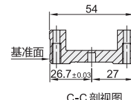
C-C 剖视图
