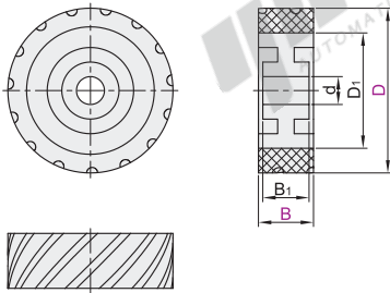
田形:主动轮 QBR75
