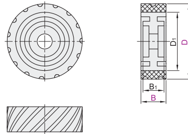
田形:从动轮 QBR76
