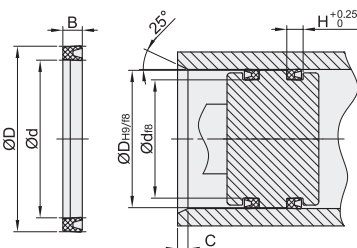
安装尺寸图a
