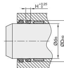
安装尺寸图b
