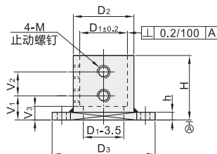
对边法兰型 RCB11/12
