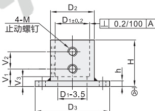
圆法兰型 RCB01/02/06
