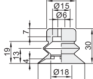
盘径 \varnothing 40
