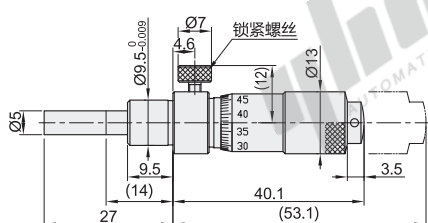
直柄型·平面测量面 EPF08-148-150(行程: 0~13)
