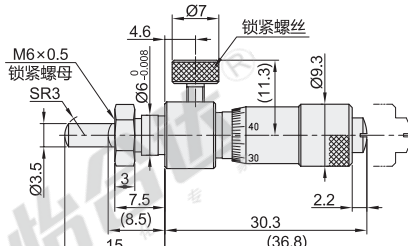
带锁紧螺母·球面测量面 EPF07-148-223(行程: 0~6.5)
