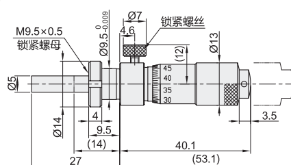
带锁紧螺母·平面测量面 EPF08-148-151(行程: 0~13)
