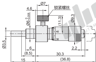
直柄型·平面测量面 EPF07-148-220(行程: 0~6.5)
