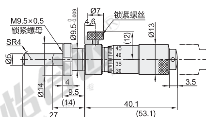
带锁紧螺母·球面测量面 EPF08-148-153(行程: 0~13)
