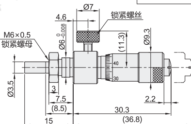
带锁紧螺母·平面测量面 EPF07-148-221(行程: 0~6.5)
