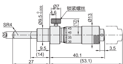
直柄型·球面测量面 EPF08-148-152(行程: 0~13)
