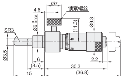
直柄型·球面测量面 EPF07-148-222(行程: 0~6.5)
