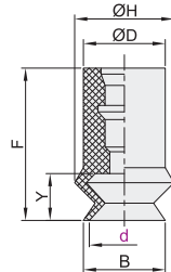
风琴形 盘径Ø6~8
