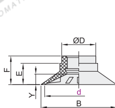
平形带肋 盘径Ø10~50
