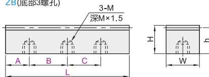
ZB (底部3螺孔)
