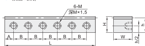
GR (侧面6螺孔)
