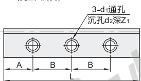
GP (侧面3沉孔)
