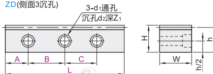
ZD (侧面3沉孔)
