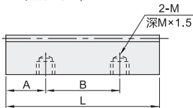
GB (底部2螺孔)
