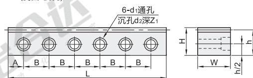
GS (侧面6沉孔)
