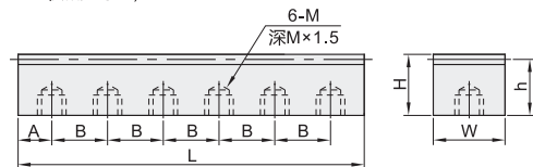
GQ (底部6螺孔)
