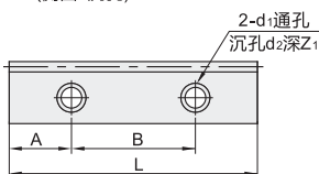
GF (侧面2沉孔)
