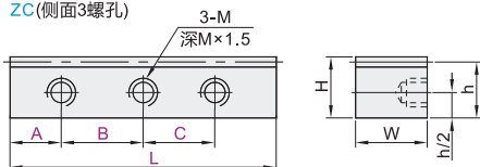
ZC (侧面3螺孔)
