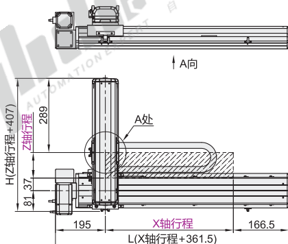
❑ X轴尺寸
