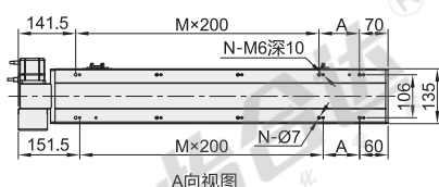
❑ X轴尺寸
