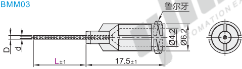
挠性 BMM03
