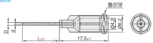
螺口型 BMM06
