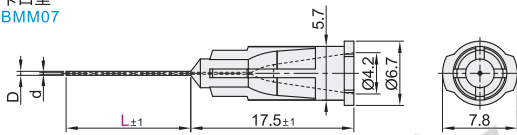
卡口型 BMM07
